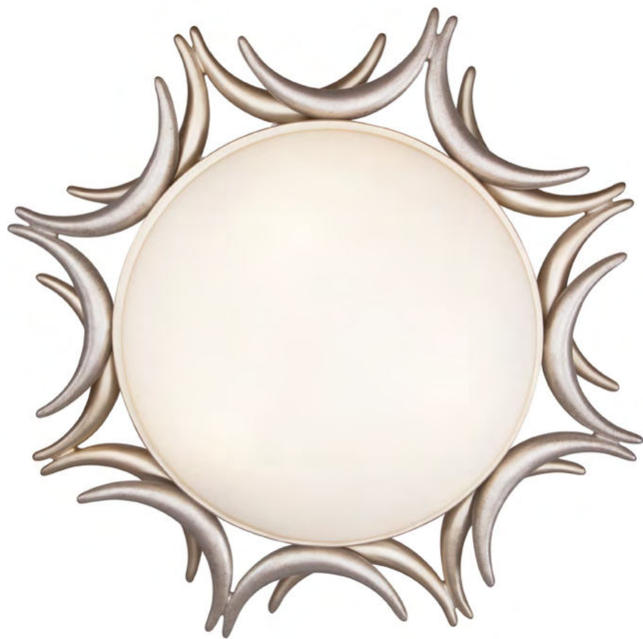
▲ H013CL-03G ⌀ 3 × E14 40W Ø430 × 115 мм △ d=260, h=80 мм
