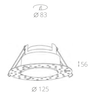
◀ DL043-01B 1 × GU10 50W 220-240 V, IP20 Ø 125 × 56 мм
