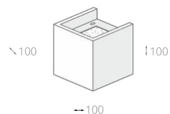
◀ C155-WL-02-3W-W LED 6W 580 lm, 3000 K, \nu , 120 ° 220-240 V, IP20 100 × 100 × 100 мм
