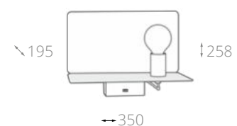
▲ C182-TL-01-B 1 × E27 60W 220-240 V, IP20 258 × 350 × 195 мм
