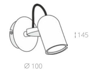
◀ SP311-CW-01-N 1 × GU10 50W 220-240 V, IP20 Ø 100 × 145 мм
